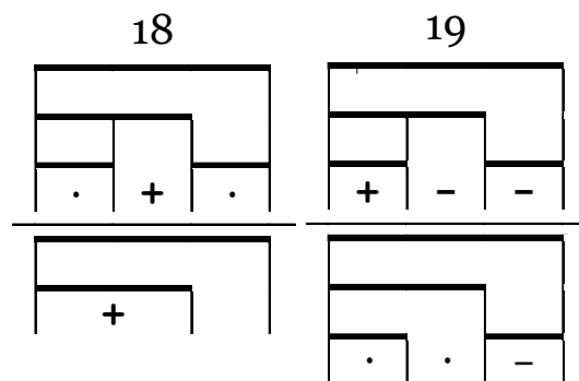
Рис. 6. Диаграммное представление правила вывода 18 и действия правил 16 и 17
