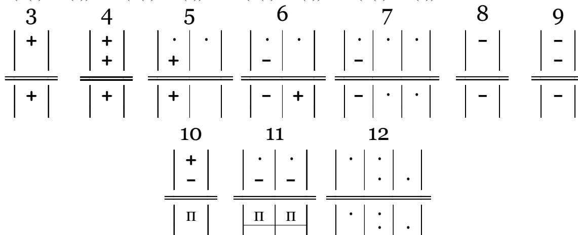
Рис. 4. Диаграммное представление правил вывода 3 и 12
